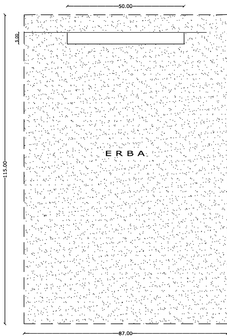
PIANTA
